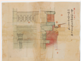
奈良博物館新築絵画室軒樋呼樋取設方拾分壺之図 (以上、「内匠寮奈良博物館建築工事図面」のうち 当館)
